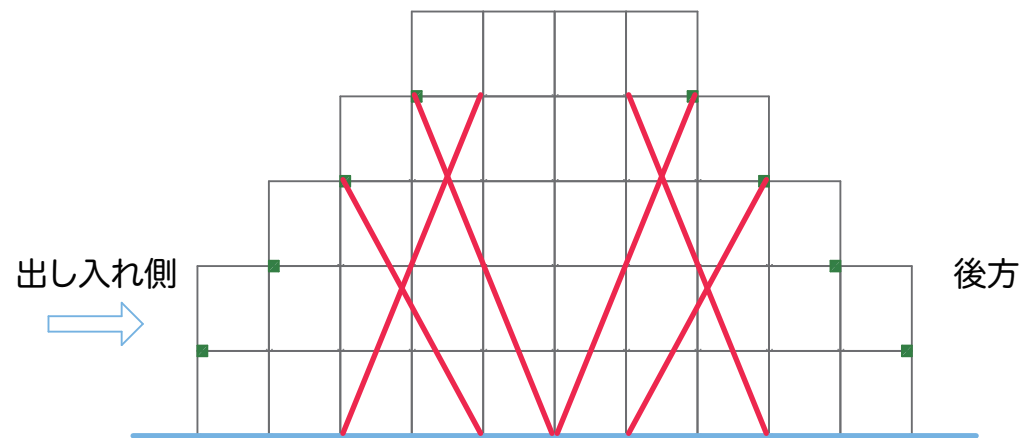
B案 ラッシング
